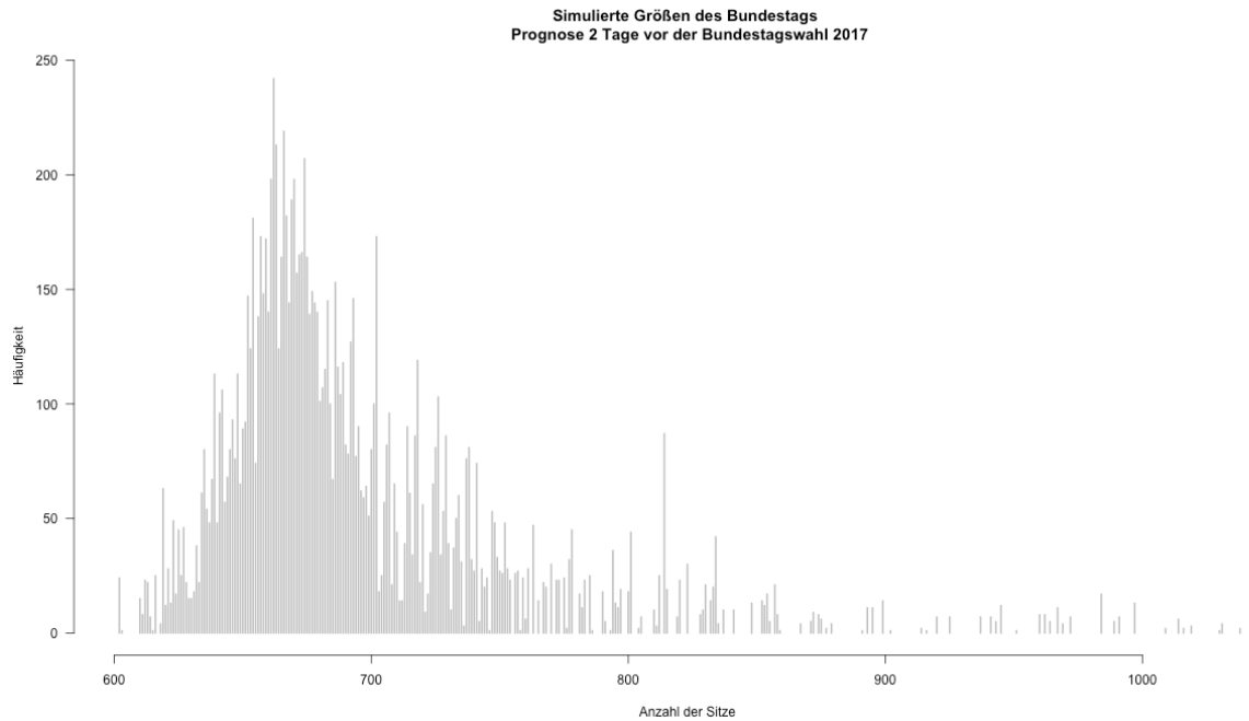
Abbildung 3: Simulierte Größen des 19. Bundestags
