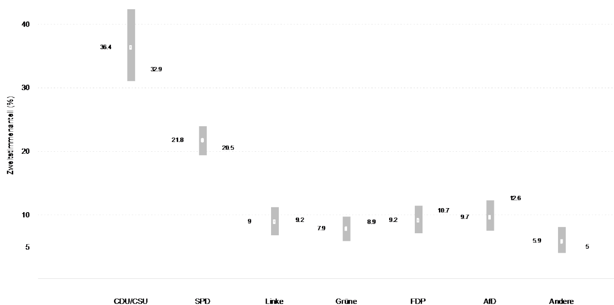
Abbildung 1: Vorhersage der Zweitstimmenanteile zwei Tage vor der Bundestagswahl 2017
